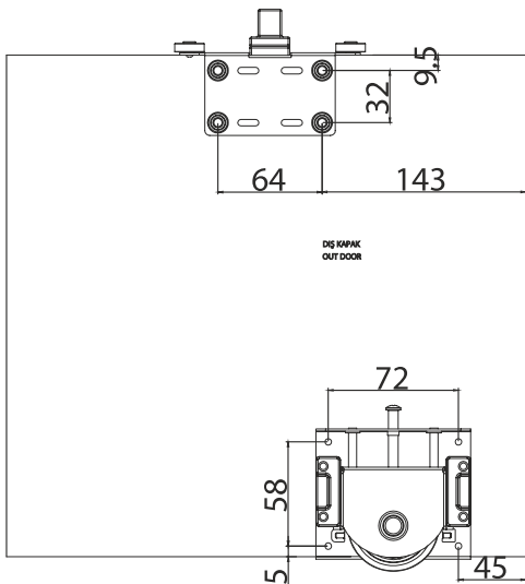
ÜST RAY
