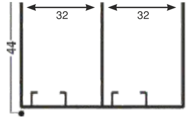
ÜST RAY
